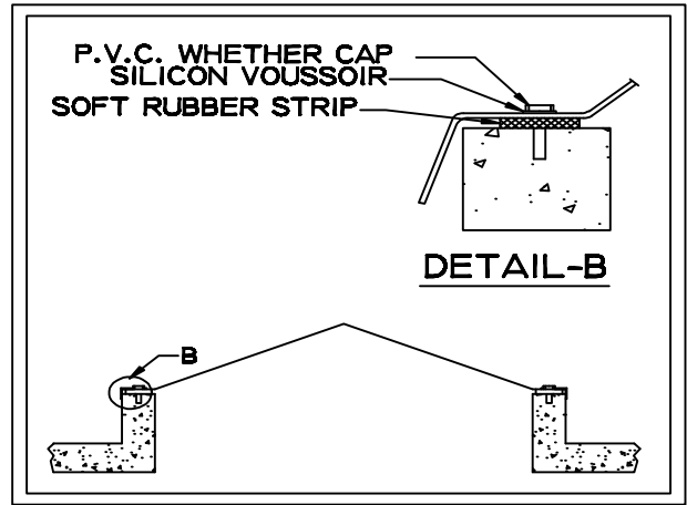
STEP FLANGE
